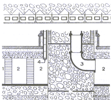
Perfil vertical del hipocausto de las Termas de Caracalla. 1, pilar de sostenimiento; 2, calefacción; 3, descarga; 4, canal de calefacción. Arriba: muro con canales de calefacción.
