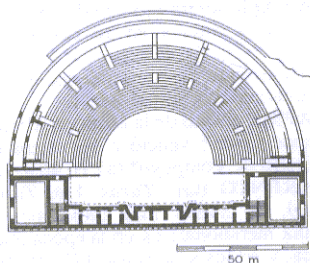
Planos del teatro griego de Epidauro (a la izquierda) y del teatro romano de Orange.
