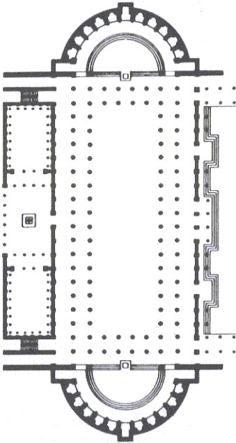
Reconstrucción de la basílica de Trajano, en Roma, concebida por Apolodoro de Damasco (principios del s. II aprox. desp. J.C.). A la izquierda: plano.
