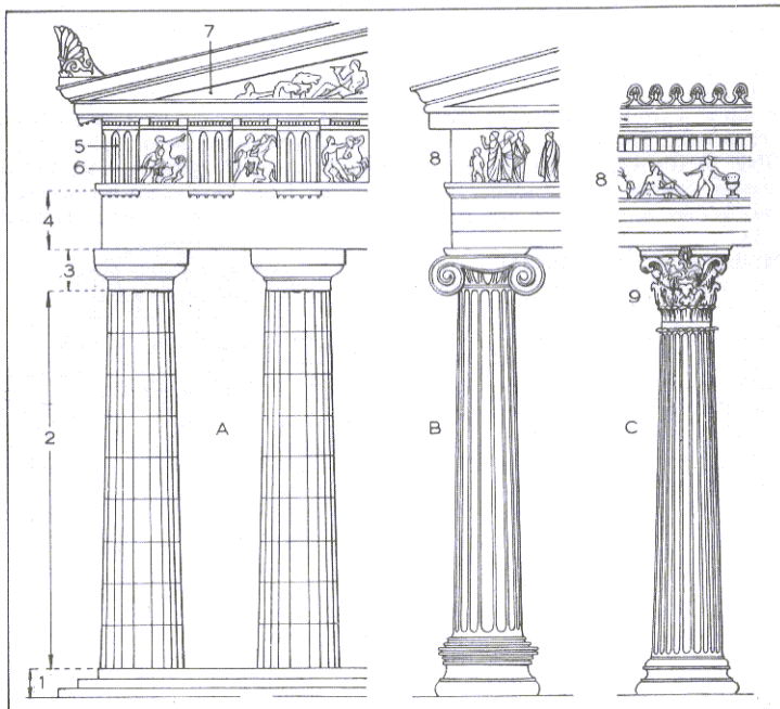
Los tres órdenes arquitectónicos griegos
