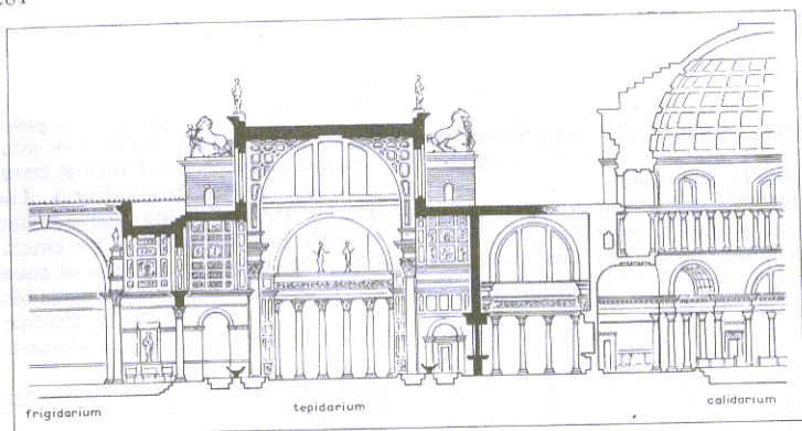
Reconstrucción de una parte de las Termas de Caracalla
